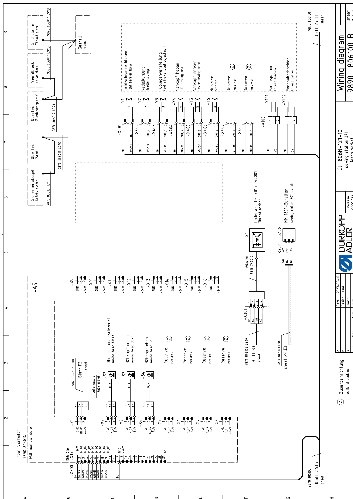
Fig. 98: Wiring diagram (8)
