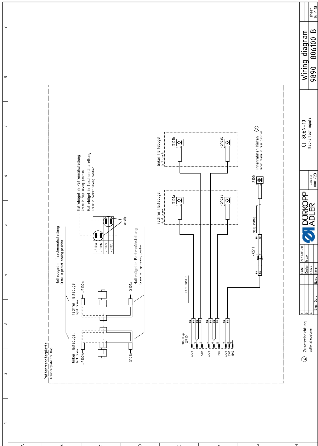
Fig. 106: Wiring diagram (16)
