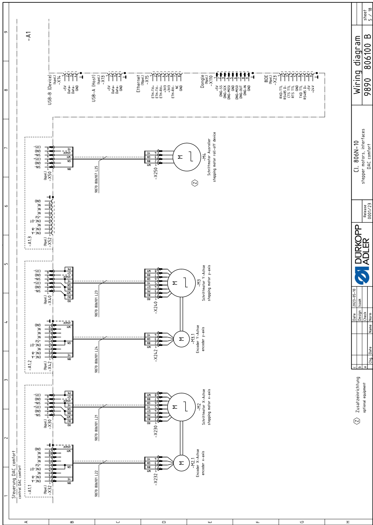
Fig. 95: Wiring diagram (5)
