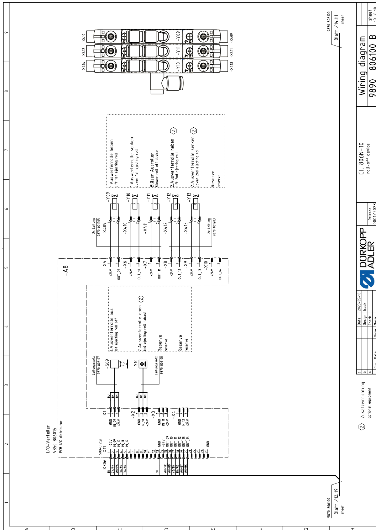
Fig. 103: Wiring diagram (13)
