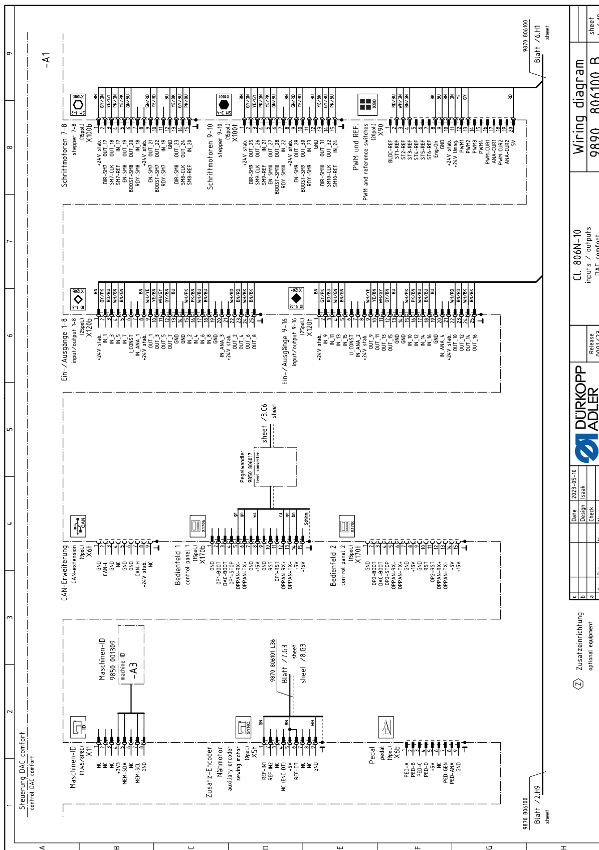
Fig. 94: Wiring diagram (4)
