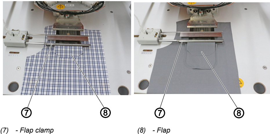
Fig. 45: Sewing (806N-521) (3)
