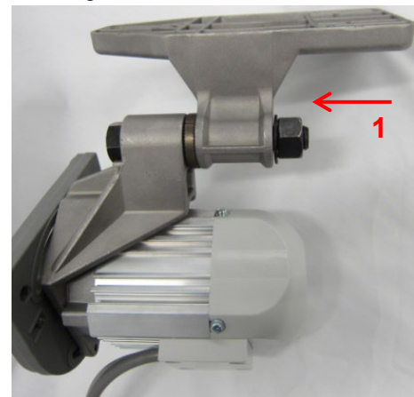
Fig. 3: Motor
