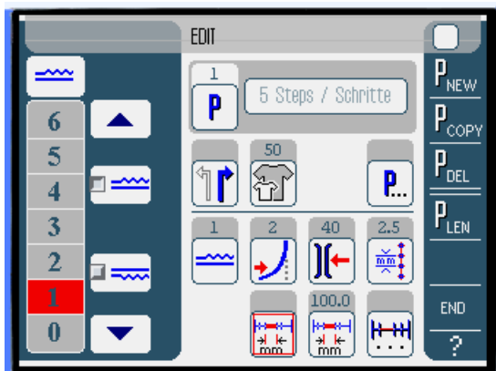
图 56： 在当前缝纫步骤中设置丰满度
