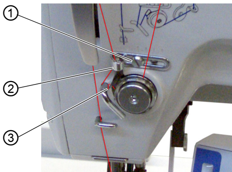
图 12：设置针线调线器
