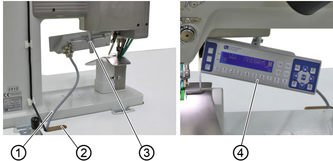
图 87：连接操作面板 OP3000
