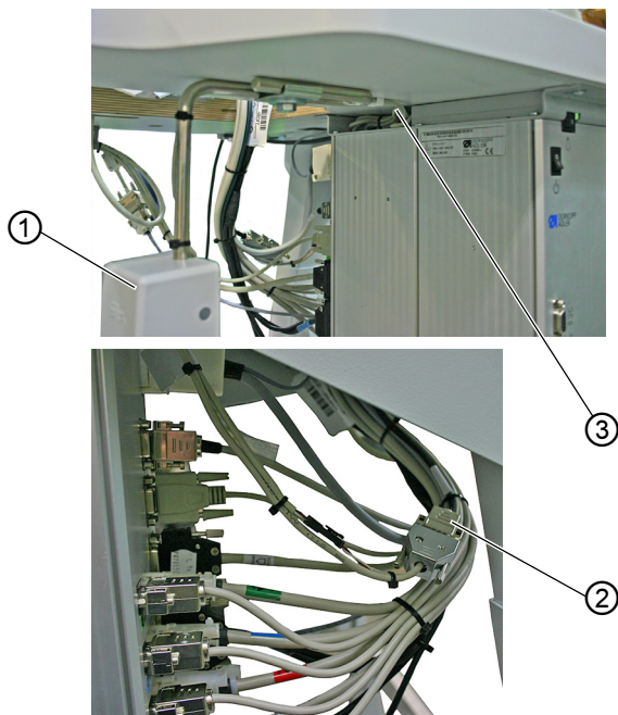
图 86：连接膝控开关
