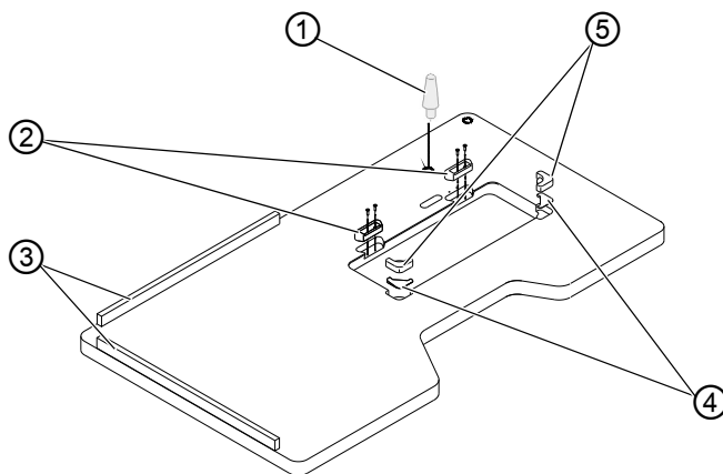
图 79 : 完成工作台板
