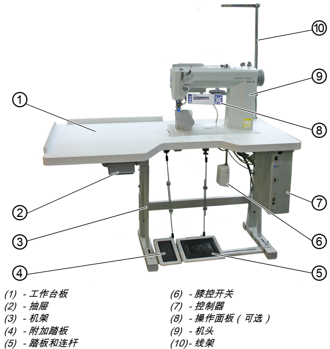
图 1: 机器组件
