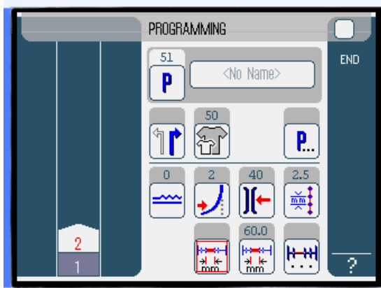
图 60：创建新的缝纫程序 (2)
