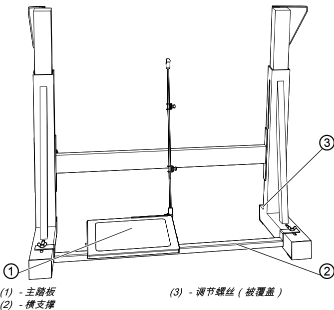
图 77：安装机架
