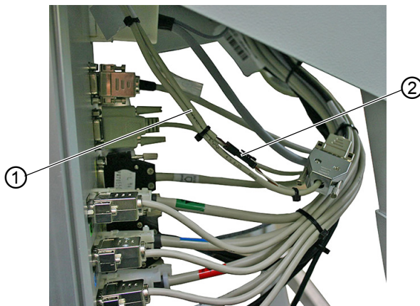
图 84：连接 LED 缝纫照明灯
