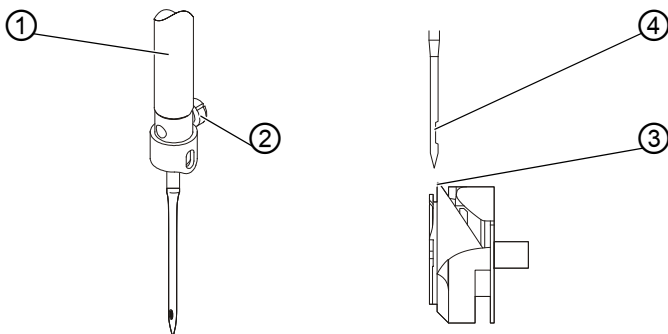
图 3：更换机针
