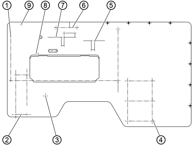
图 78：预装工作台板
