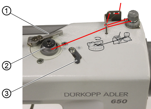
图 6：绕梭芯线
