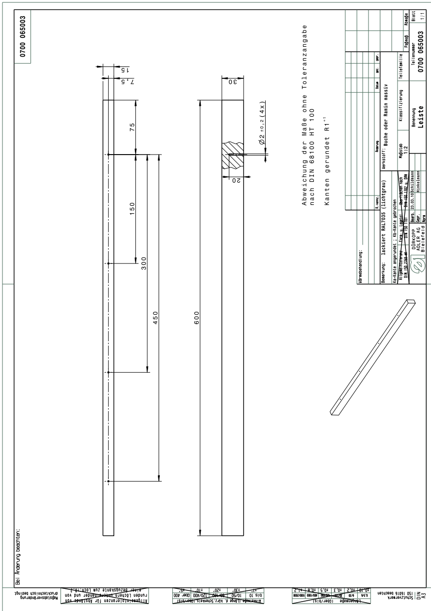
图 92：用于制造工作台板的尺寸
