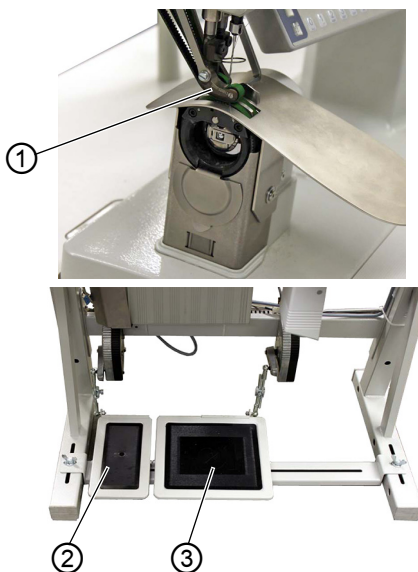
图 13：抬起缝纫压脚
