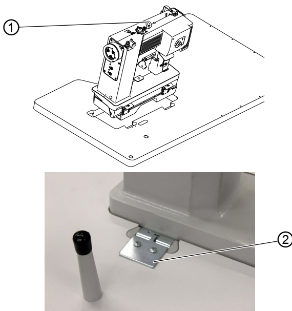
图 82：装入机头
