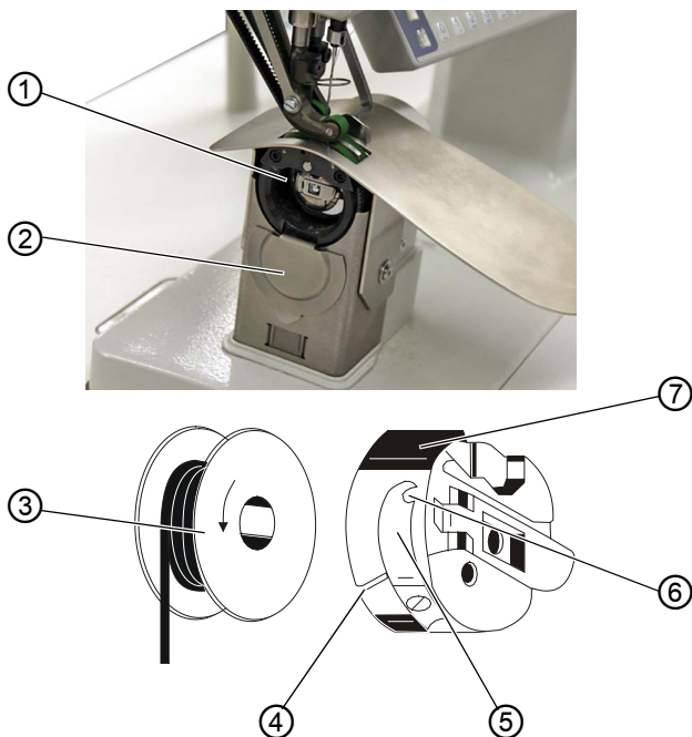
图 7：更换梭芯
