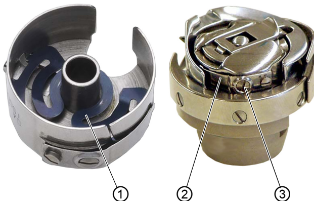
图 11：设置梭芯线张力 (2)
