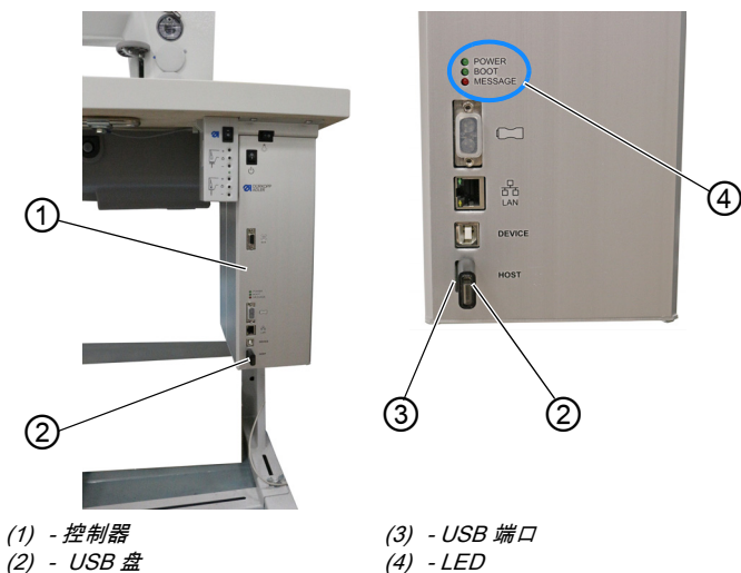
图 41：执行软件更新
