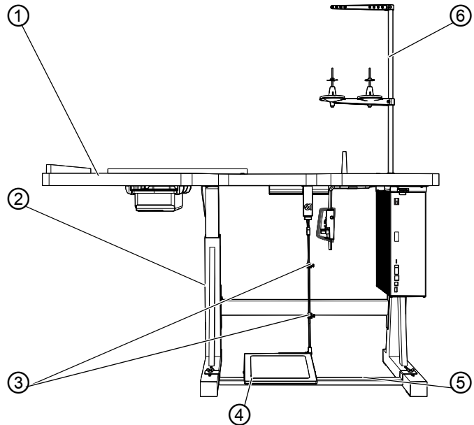
图 80：固定工作台板和踏板
